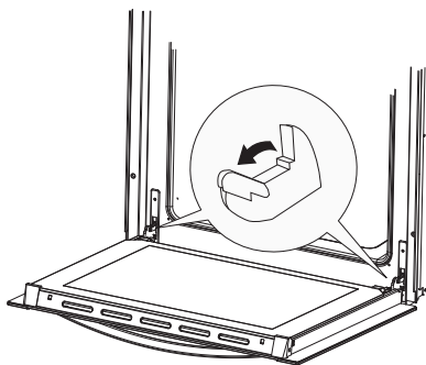
Установка защелки предохранителя
