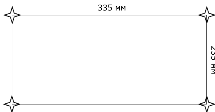
Рисунок 7 – Расстояние для сверления отверстий (монтаж на стену)
