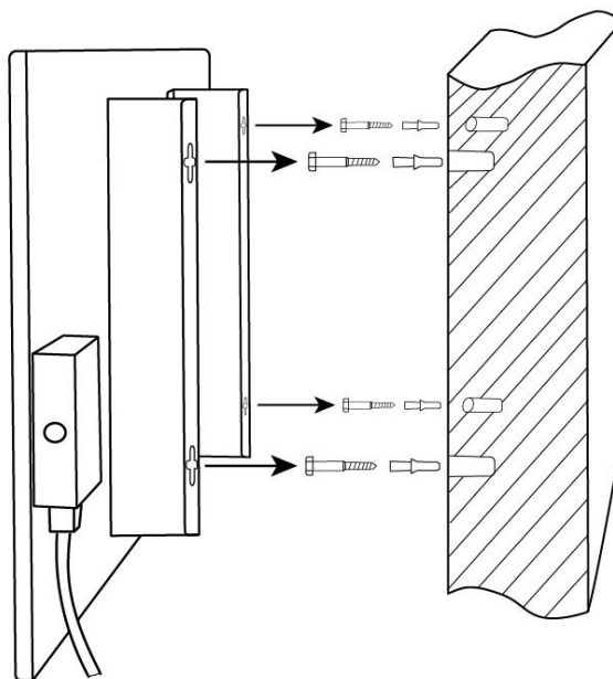
Рисунок 6 – Монтаж на кронштейны (на стену)
