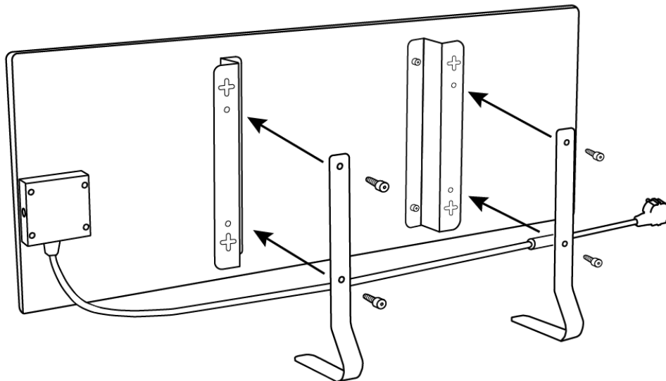
Рисунок 5 – Монтаж на ножки (на пол)
