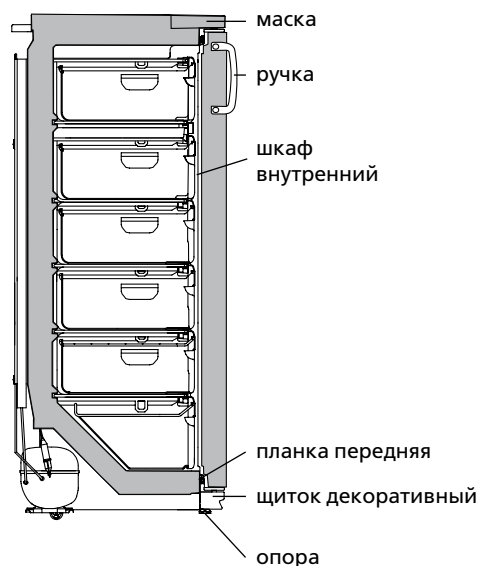
Рисунок 6 – Схема морозильника
