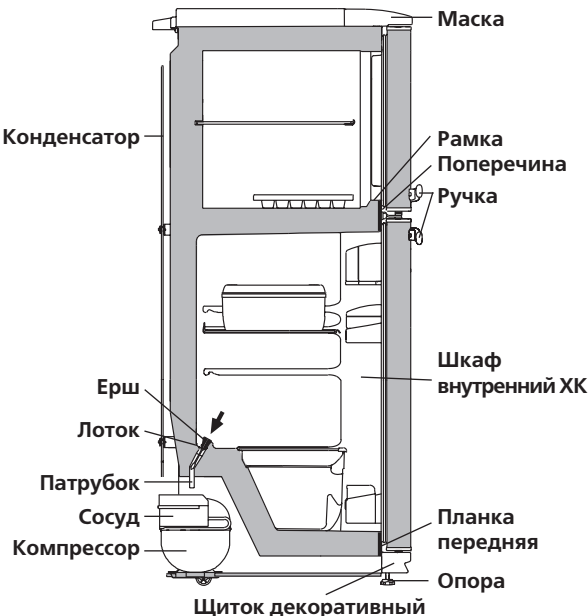
Рисунок 7 — Схема слива талой воды
