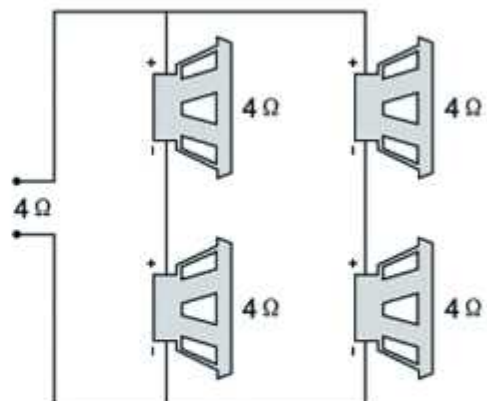
Последовательно-параллельное подключение
