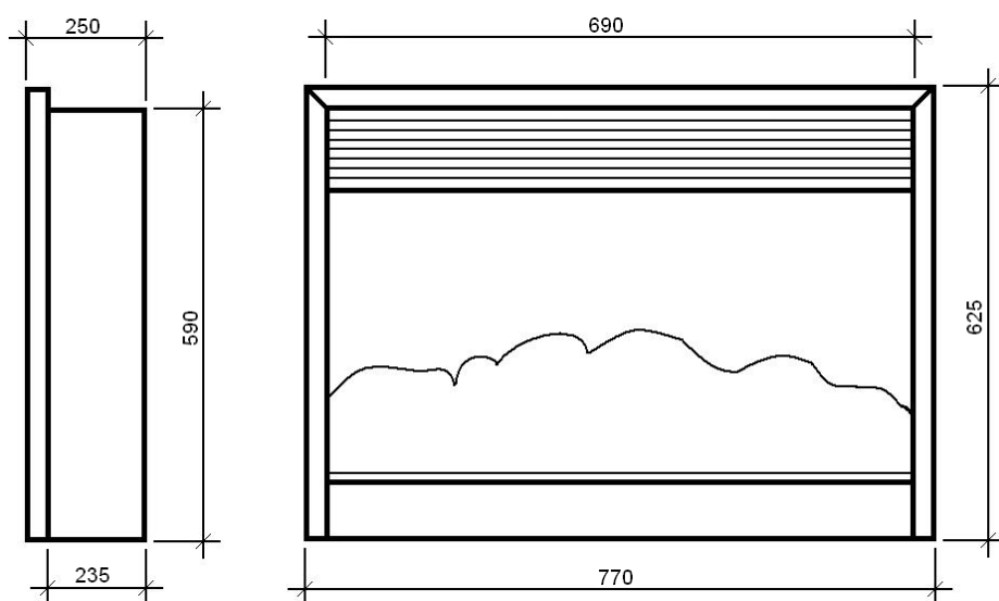
Рис. 1. Внешние размеры указаны для A01BL1FX
