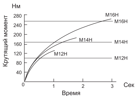
Усиленный крепеж
