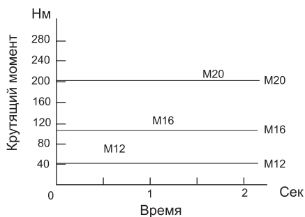
Стандартный крепеж
