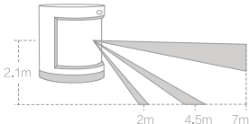
유효 감지 영역 - 측면도
