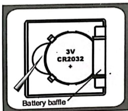
Battery baffle – щиток батареи РИС. 1
