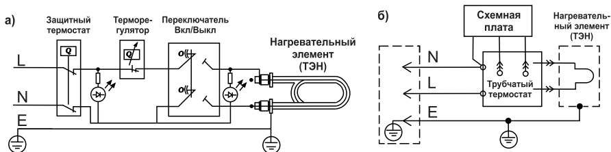
Рис. 4 Принципиальная электрическая схема водонагревателя: а) «WH» модели, б) «TT WH» модели
