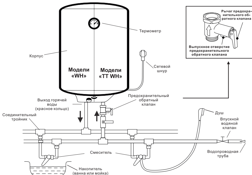
Рис. 1 Общая схема водонагревателя, подключенного к водозаборной точке
